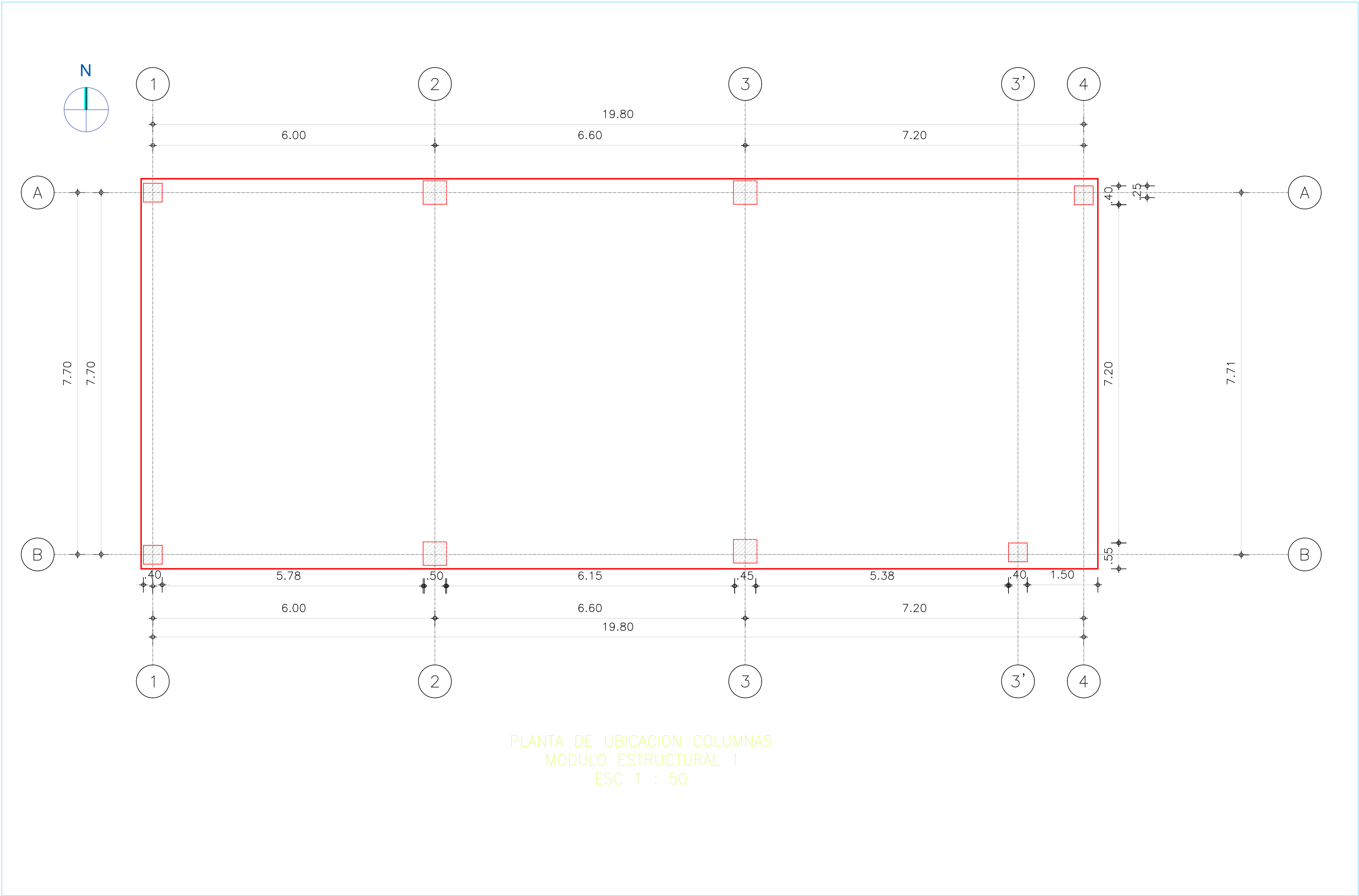
DESPIECE DE COLUMNAS –MODULO ESTRUCTURAL 1–
