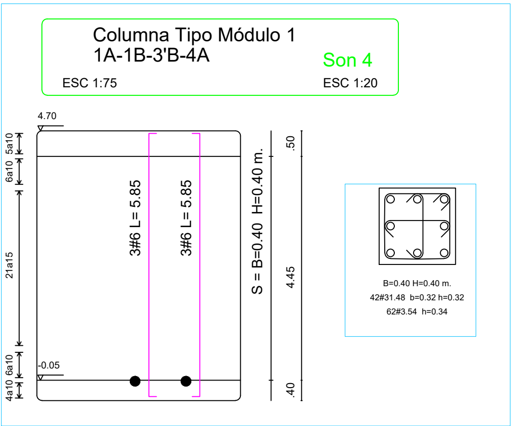
DESPIECE DE COLUMNAS –MODULO ESTRUCTURAL 1–
